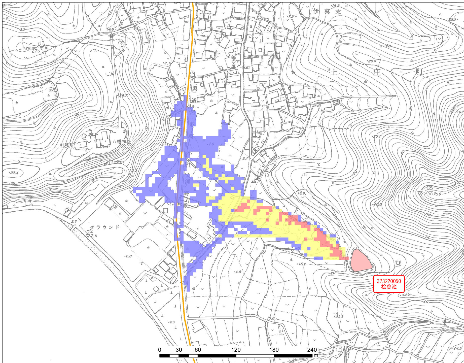
土庄町ため池氾濫解析 浸水想定区域図 (歩行困難区域)
